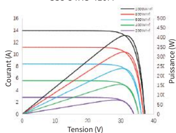
Courbe courant/puissance - tension SS8-54HS-410M
