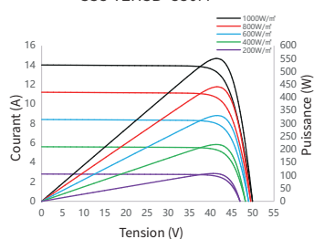
Courbe courant/puissance - tension SS8-72HSB -550M
