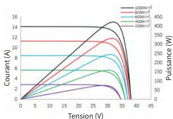
Courbe courant/puissance - tension SS8-54HD-420N
