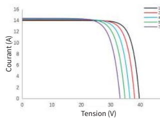
Courbe courant - tension SS8-54HD-420N
