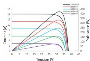
Courbe courant/puissance - tension SS8-54HDB-420N
