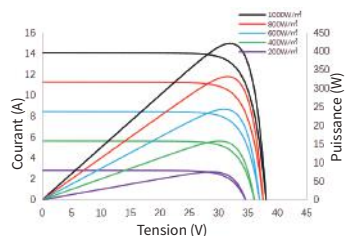
Courbe courant/puissance - tension SSA-48HD-445N
